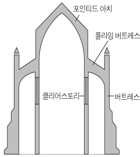
고딕 성당의 단면도
